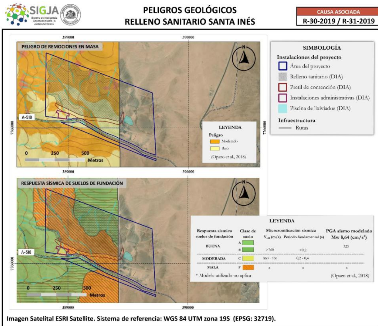
Mapa 2. Peligros Geológicos en el sector del proyecto Relleno Sanitario Santa Inés: peligro de remociones en masa y respuesta sísmica de suelos de fundación. Fuente: Primer Tribunal Ambiental, en base a Mapas 2 y 3 de Carta de Peligros geológicos del área de Iquique-Alto Hospicio, Región de Tarapacá (Opazo et al., 2018) y expediente de evaluación ambiental.
