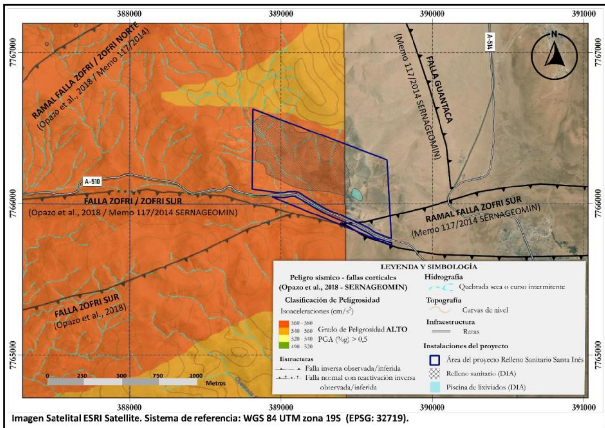
Mapa 1. Peligro sísmico asociado a fallas cuaternarias. Fuente: Primer Tribunal Ambiental, en base a Mapa 4 de Carta de Peligros geológicos del área de Iquique-Alto Hospicio, Región de Tarapacá (Opazo et al., 2018), Memo 117/2014 de SERNAGEOMIN y expediente de evaluación ambiental.
